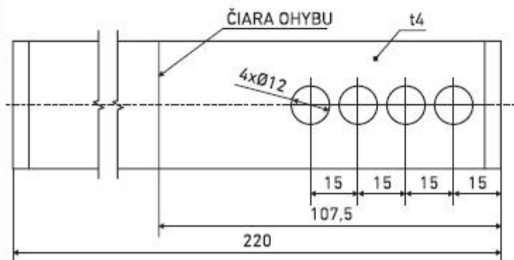
ROZVINUTÝ POHLAD
